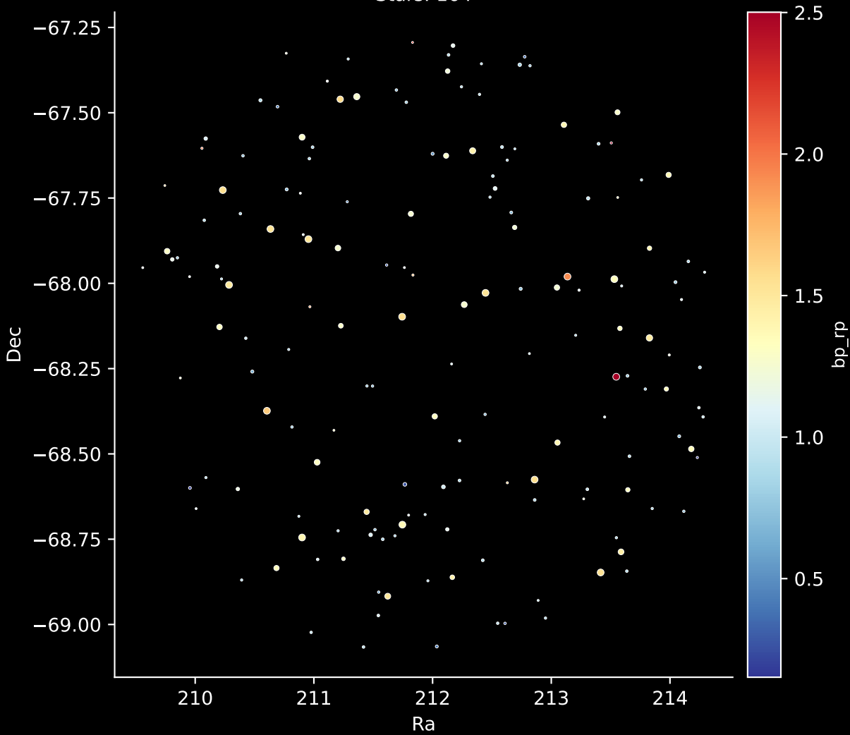
APOGEE DR17 Field: [280-22-O_TESS] Stars: 164
