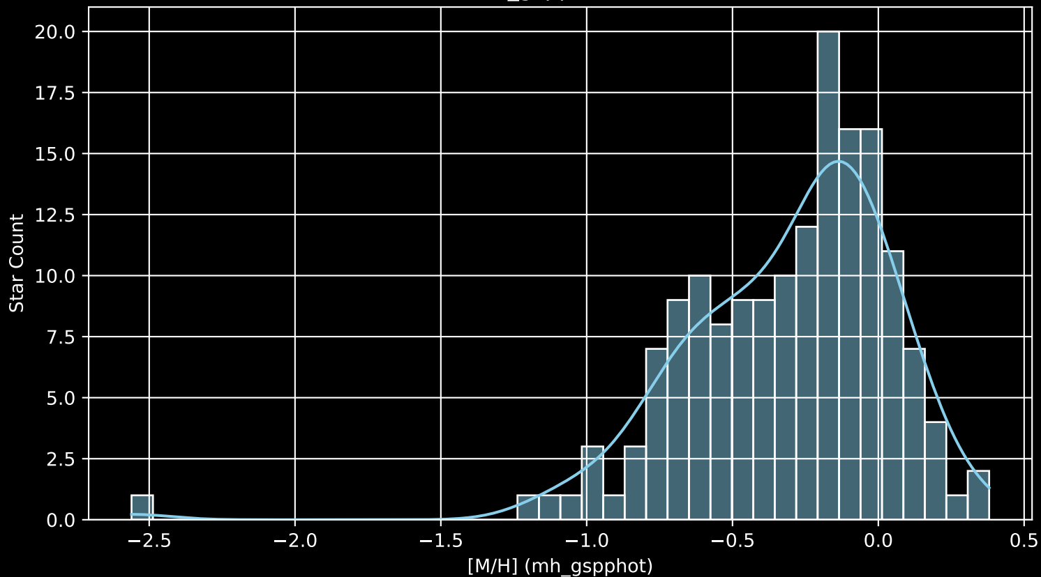
APOGEE DR17 Field: [280-22-O_TESS [M/H] (mh_gspphot) (n= 162)
