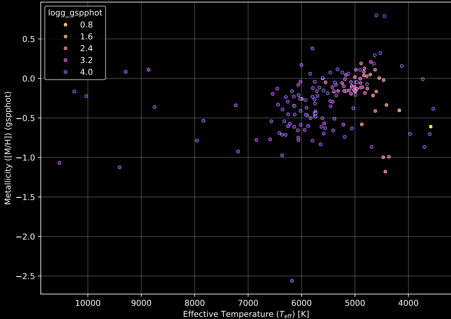
APOGEE DR17 Field: [280-22-O_TESS] Stellar Population Parameters (n= 164)
